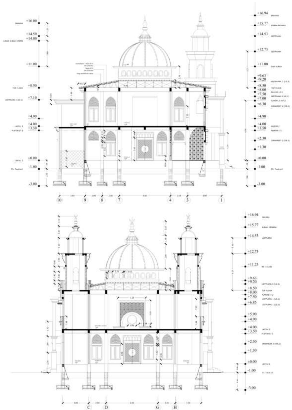
[Gambar 2. Tampak dan Perspektif Masjid]
